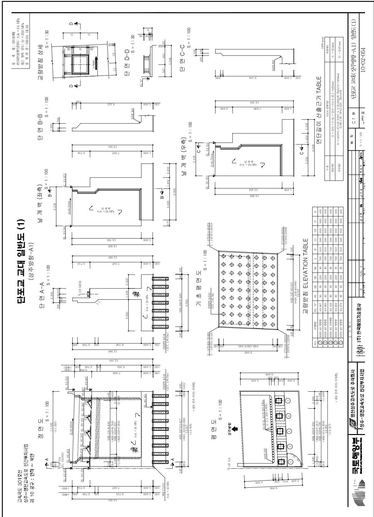
【그림 28.1.8】 교대 일반도(상주방향)
